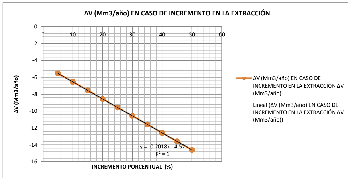
Gráfica 9. \Delta v (mM 3 /AÑO) en caso de incremento en la extracción porcentualmente con base a la extracción actual de 20.18 (mM 3 /Año)
