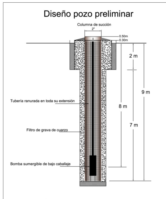
Figura 6.1 Diseño constructivo de pozos de extracción.
