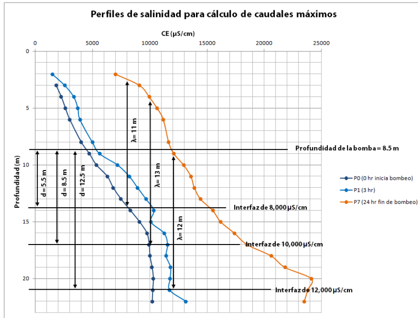
Figura 5.36 Interfaces establecidas en los perfiles de salinidad de la prueba de bombeo.
